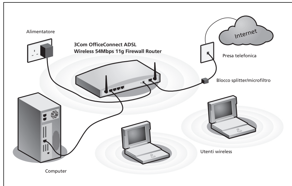
Esempio di rete con 3Com OfficeConnect ADSL Wireless 54 Mbps 11g Firewall Router
